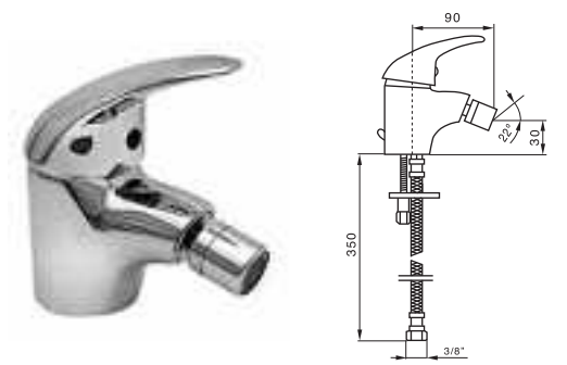
44.009 Monomando bidé Bidet mixer Mitigeur bidet Einhebel bidetmischer Однорычажный Смеситель для Биде
