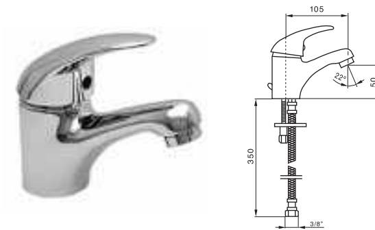
44.002 Monomando lavabo Wash-basin mixer Mitigeur lavabo Einhebel waschtischmischer Однорычажный Смеситель для раковины
