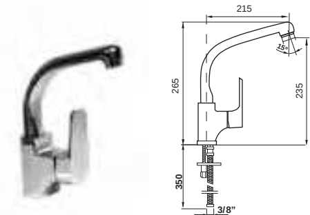
64.103 ● Monomando lavabo giratorio Basin mixer swivel spout Mitigeur lavabo avec bec orientable Einhebel Waschtischmischer Однорычажный Смеситель для раковины
