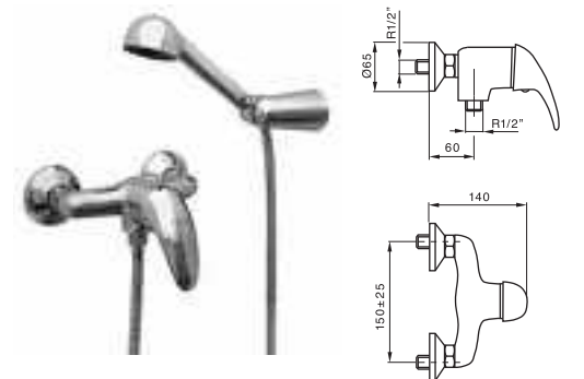
44.015 Monomando ducha con accesorios Shower mixer with accessories Mitigeur douche avec ensemble de douche Einhebel duschmischer mit Zubehör Однорычажный Смеситель для душа с аксессуарами
