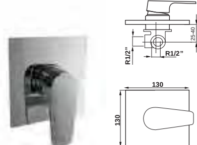
64.315 ● Monomando empotrar ducha Built-in shower mixer Ensemble douche à encastrer Unterputz duschmischer Однорычажный Смеситель встроенный для душа
