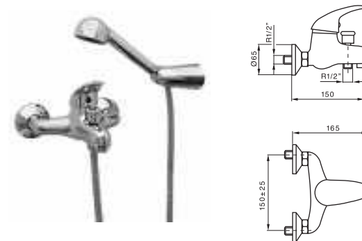
44.012 Monomando baño ducha con accesorios Bath and shower mixer with accessories Mitigeur bain-douche avec accessoires Einhebel wannen und duschmischer mit Zubehör Однорычажный Смеситель для ванны и душа с аксессуарами
