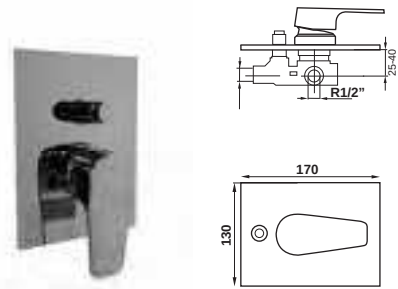
64.312 ● Monomando empotrar baño ducha Built-in bath/shower mixer Mitigeur bain-douche à encastrer Unterputz wannen und duschmischer Однорычажный Смеситель встроенный ванна душ
