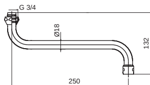
17.S25 Tubo S 25 cm Tube S 25 cm Bec tube S 25 cm Rohrauslauf S 25 cm Труба S 25 cm
