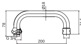
17.U20 Tubo U 15 cm Tube U 15 cm Bec tube U 15 cm Rohrauslauf U 15 cm Труба U 15 cm
